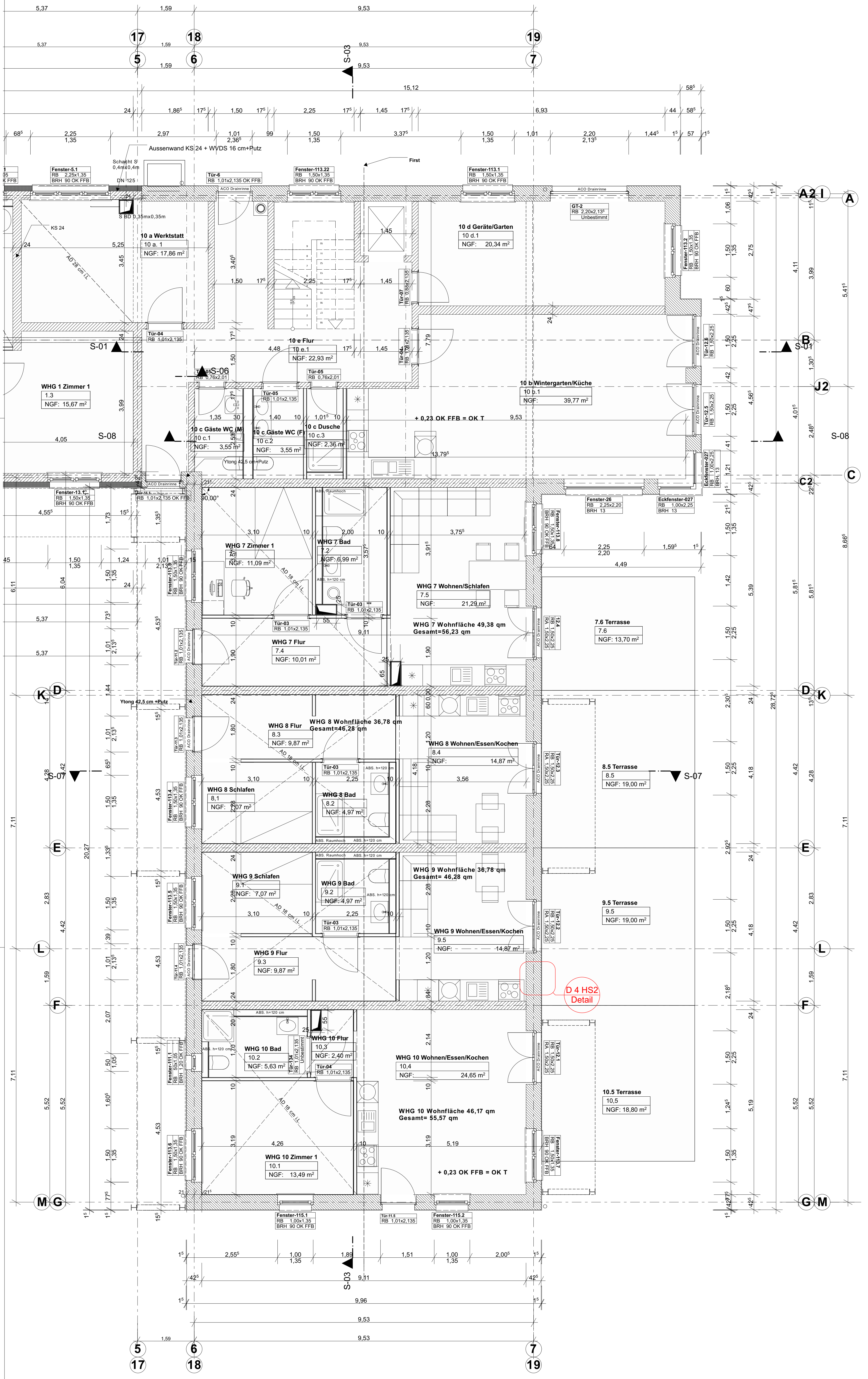
0. EG 1:50
