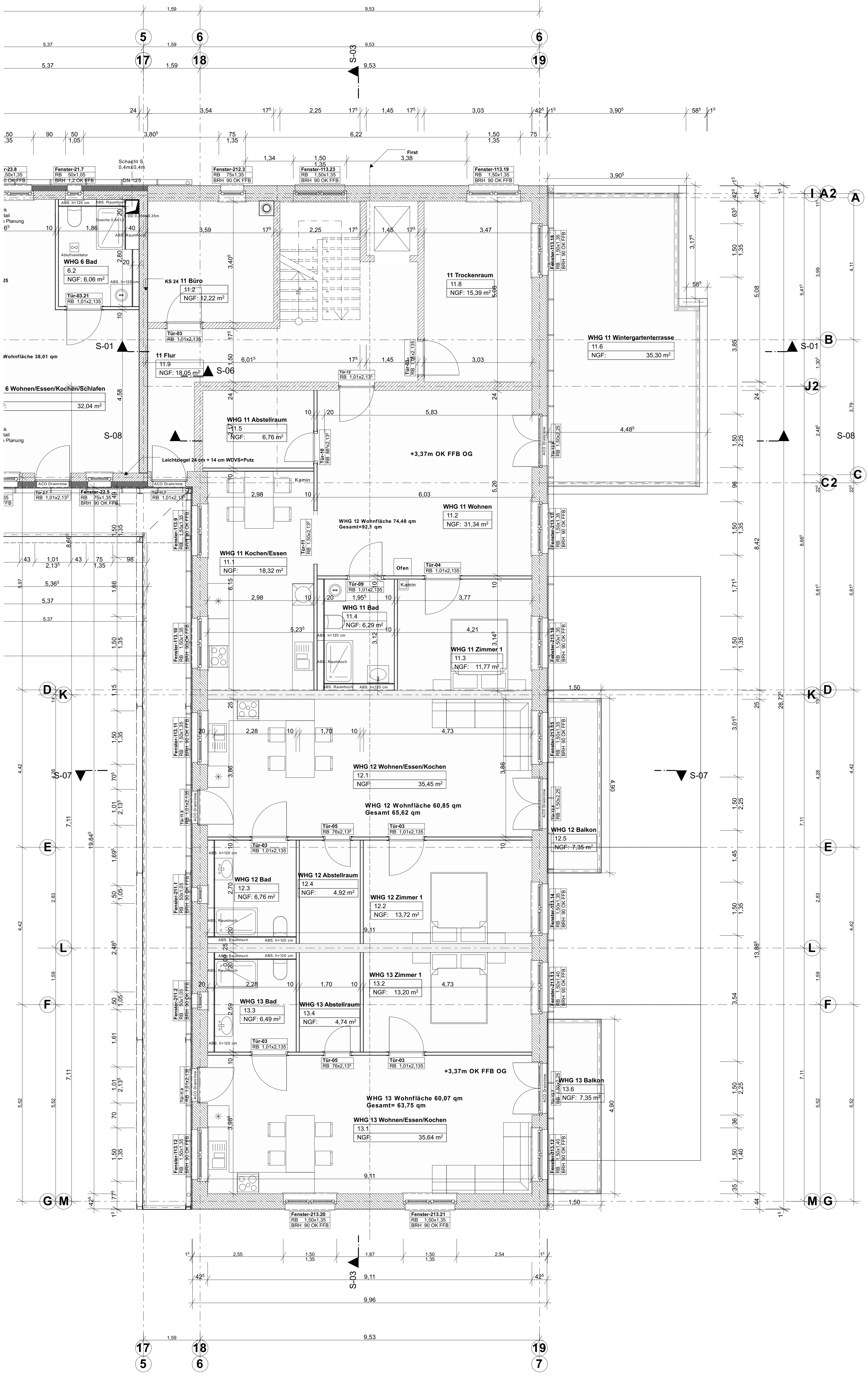
1. 1. OG 1:50
